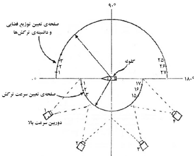
شکل ۷: نمونه‌ای از یک طراحی میدان ترکش‌گیری
