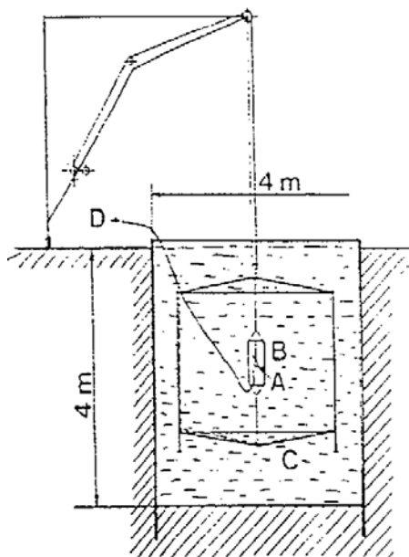
شکل ۱۳: روش ترکش‌گیری زیر آب [۱۹ و ۲۷]
