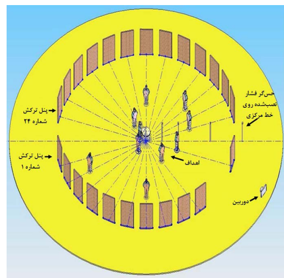
شکل ۶: چیدمان صفحات و اهداف در یک میدان ترکش‌گیری
