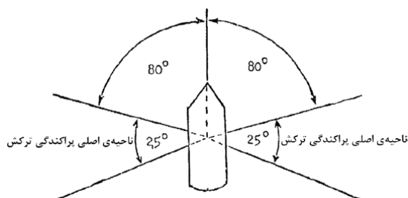
شکل ۱: نواحی اصلی پخش ترکش‌های حاصل از انفجار گلوله‌های شدیدالانفجار [۱۰]
