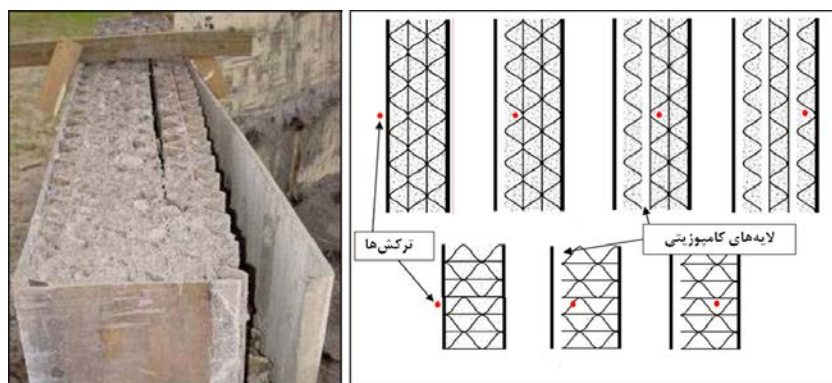
شکل ۴: نمایی از صفحات کامپوزیتی ترکش‌گیری
